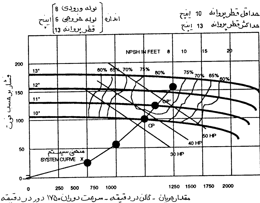
شکل ۶-۳ منحنی سیستم
