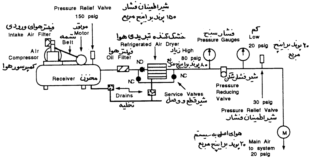
شکل ۱-۱۳ سیستم هوای فشرده با فشار منفرد
