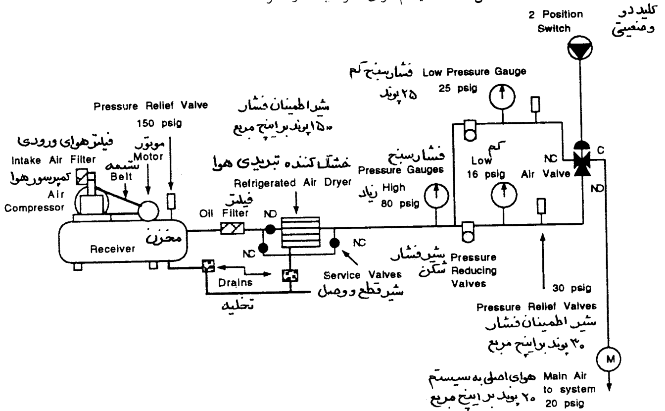
شکل ۲-۱۳ سیستم هوای فشرده دو گانه
