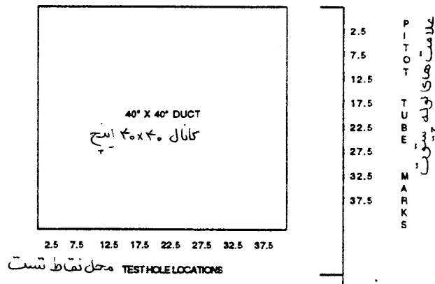
شکل ۲۰-۱۷ محل سوراخهای آزمایش دستگاه هوارسان شماره AHU-024 و علامت گذاری لوله پیتوت (کانال اصلی)
