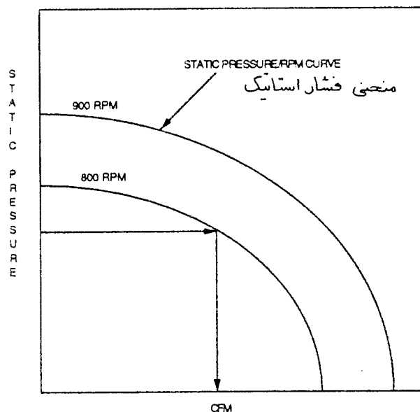
شکل ۳-۲ تعیین مقدار هوادهی (cfm) با داشتن فشار استاتیک
